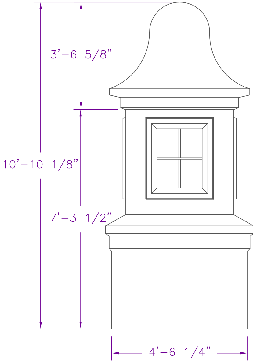
1 E1 ELEVATION
