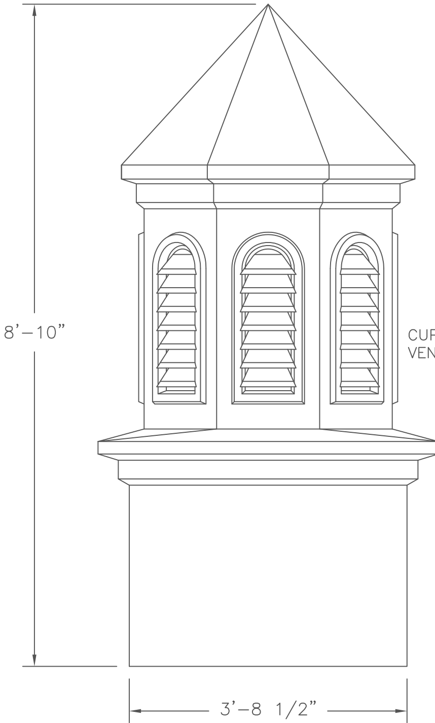
① ELEVATION
