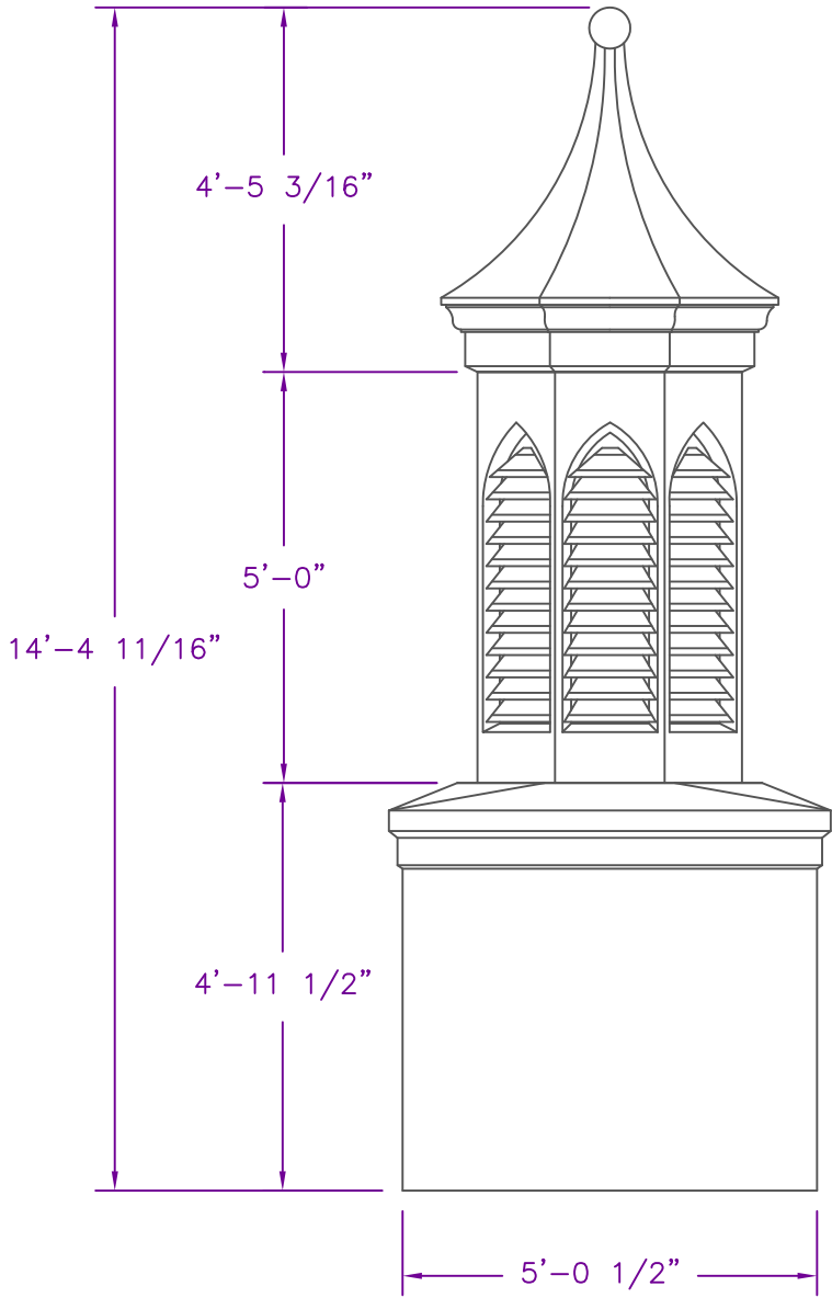
1 E1 ELEVATION
