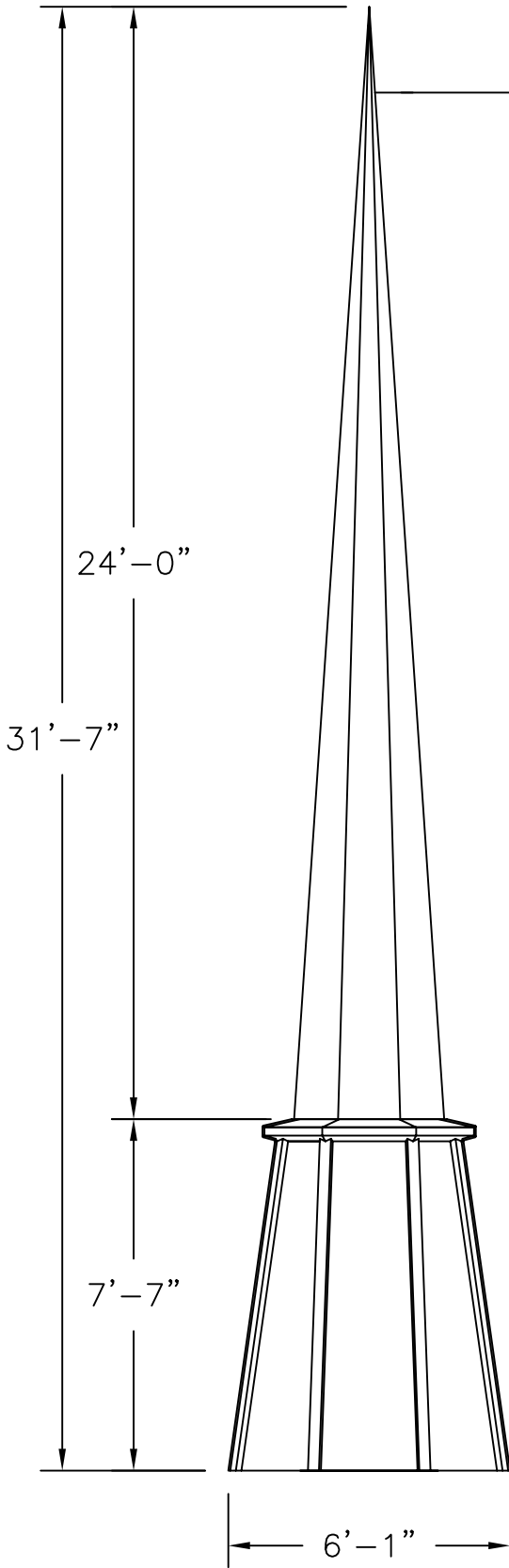
① ELEVATION E1
